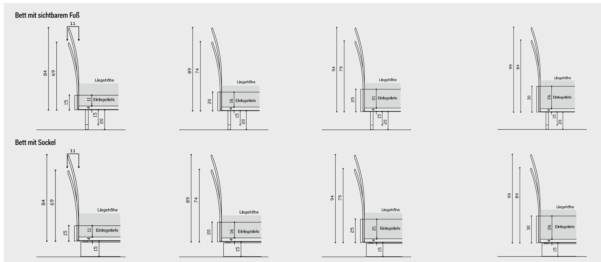
Bett mit Füßen oder Sockel mit gewölbttem Kopfteil – Maße in cm, A = Innenmaß
