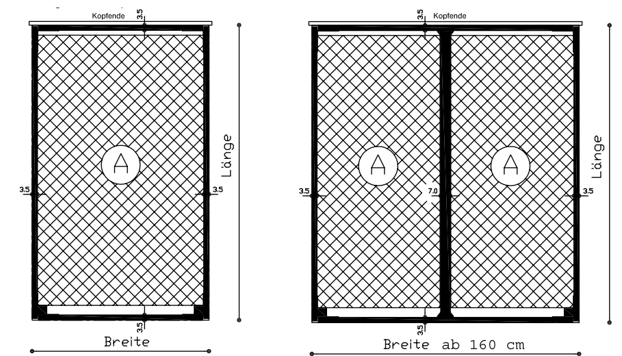
Bett mit Füßen oder Sockel mit geradem Kopfteil - Maße in cm, A = Innenmaß
