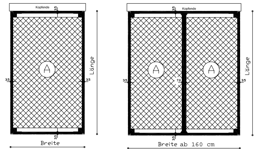
Bett mit Füßen oder Sockel mit gewölbttem Kopfteil – Maße in cm, A = Innenmaß
