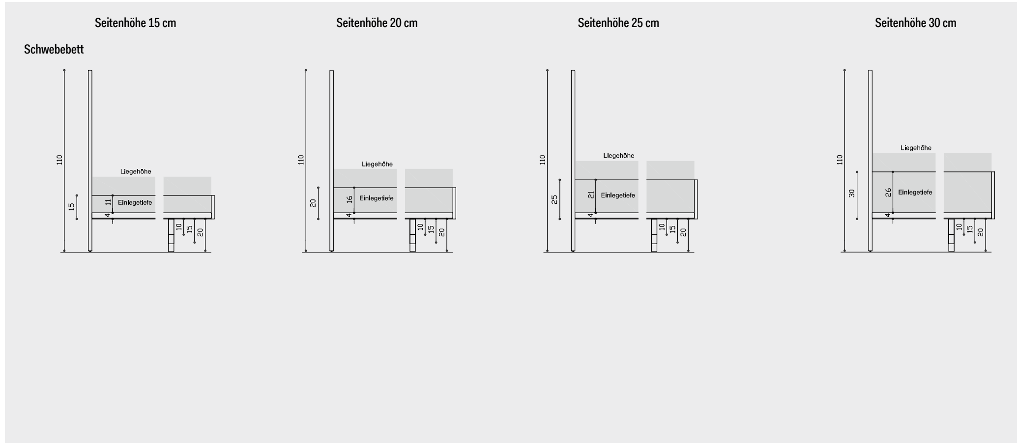
Bett schwebend mit geradem Kopfteil - Maße in cm, A = Innenmaß
