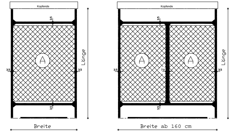
Schwebbett mit gewölbttem Kopfteil – Maße in cm, A = Innenmaß
