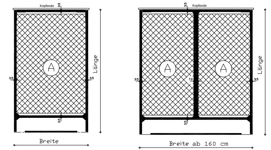
Bett schwebend mit geradem Kopfteil - Maße in cm, A = Innenmaß
