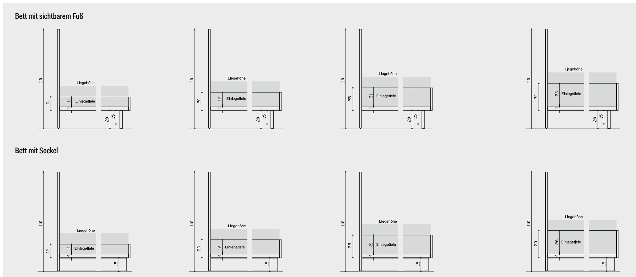
Bett mit Füßen oder Sockel mit geradem Kopfteil - Maße in cm, A = Innenmaß
